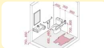
Приклад облаштування санітарно-гігієнічного приміщення (розміри вказані у мм)
